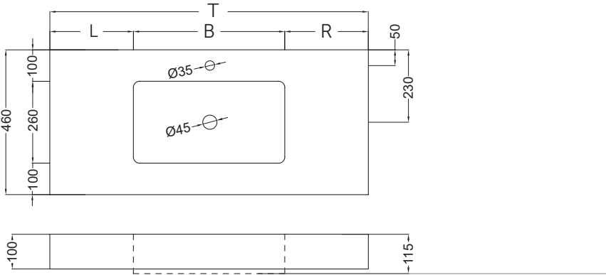
Washbasin Toren cube 60 - 200
