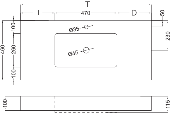
Waschtisch Toren cube 60 - 200
