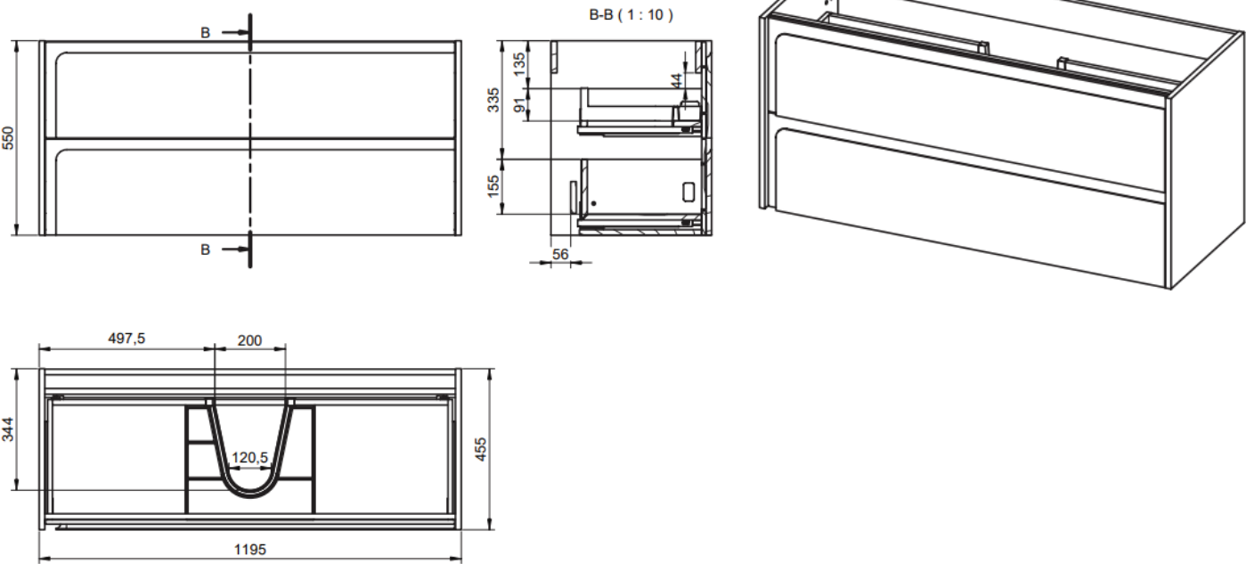
Width 120
